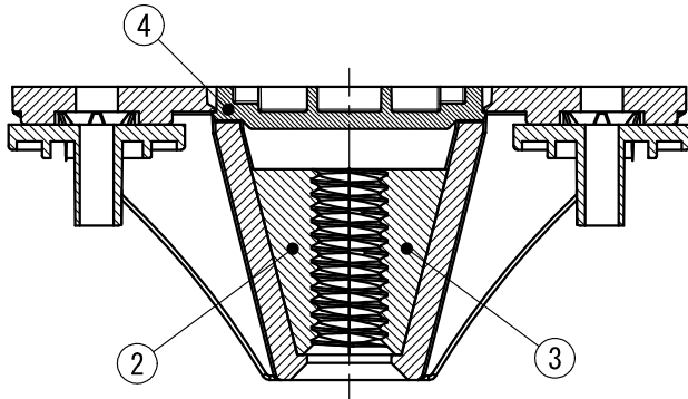
断面 A-A
